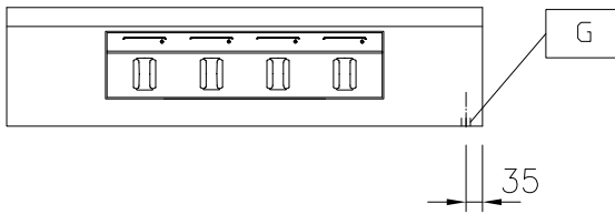
Alzado
